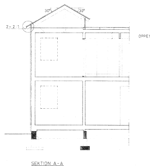
SEKTION A-A
