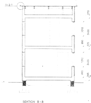
SEKTION B-B
