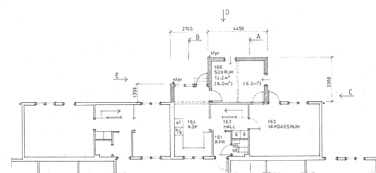
BOTTENVÅNING VID TYP C-1 ENDAST BV
