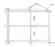
SEKTION A
