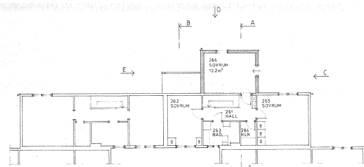
ÖVERVÅNING
